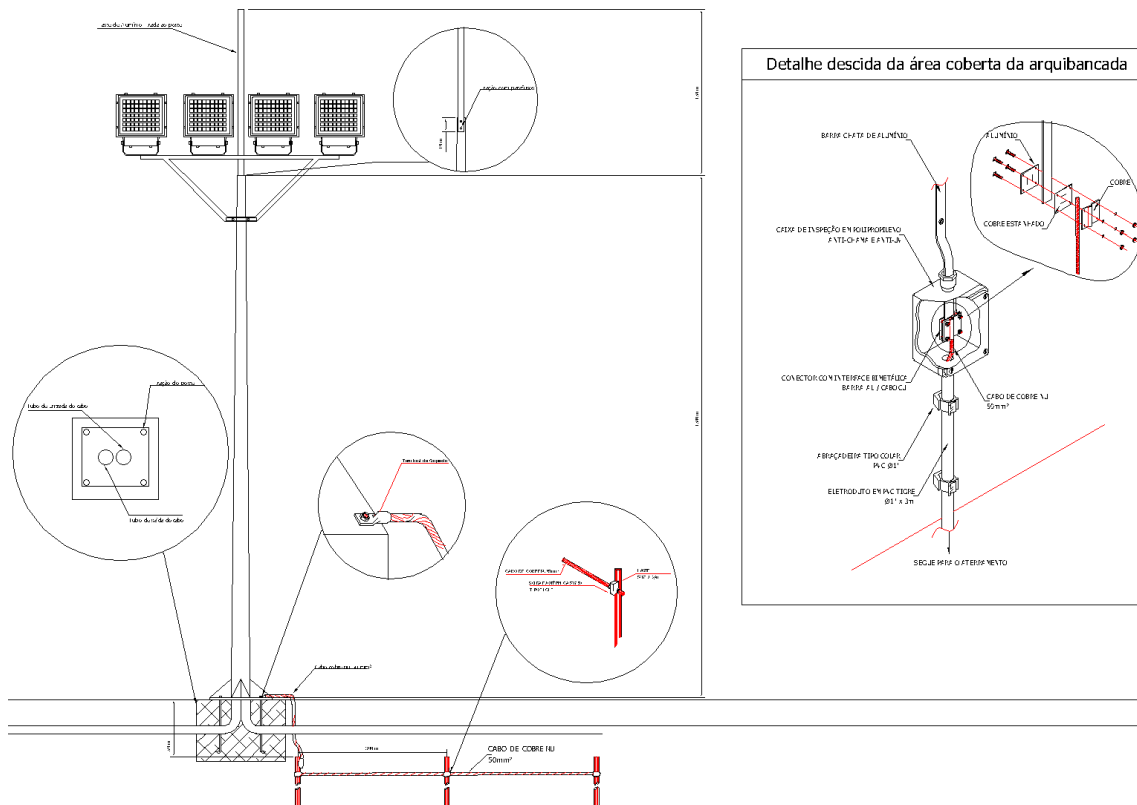
Figura 3 – Detalhe ligações Campo 1
